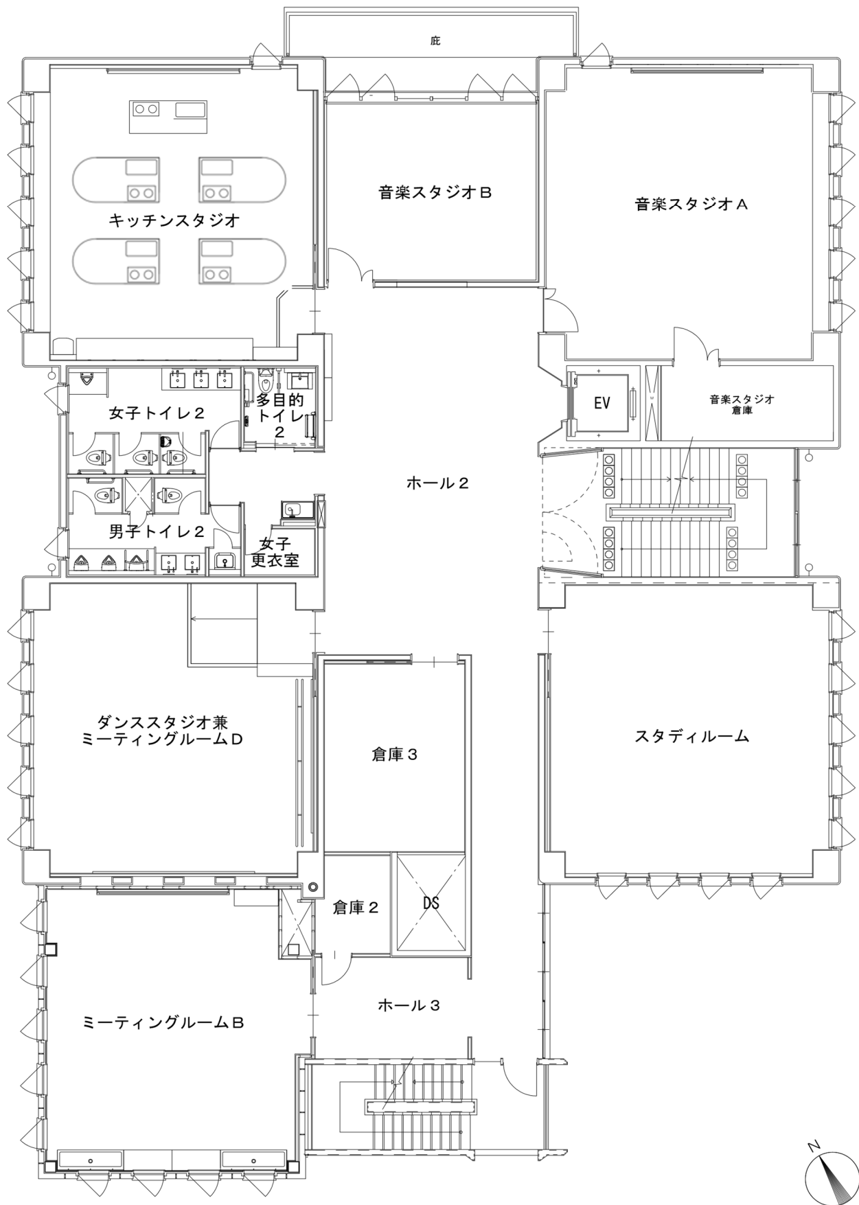
多目的棟2階平面図
